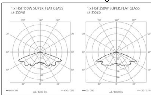
Křivka svítivosti:
