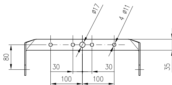
HORQUILLA FIJACION
