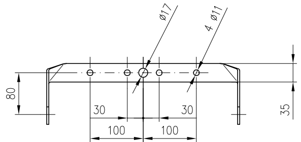
HORQUILLA FIJACION
