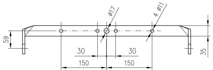
HORQUILLA FIJACION
