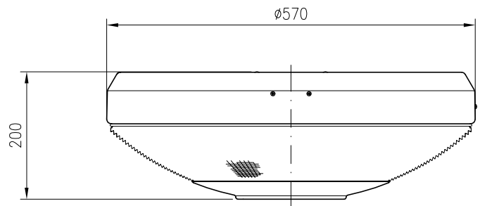
ALZADO
