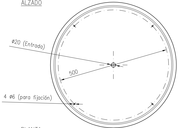
PLANTA
