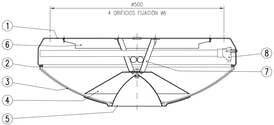
SECCIÓN TRANSVERSAL
