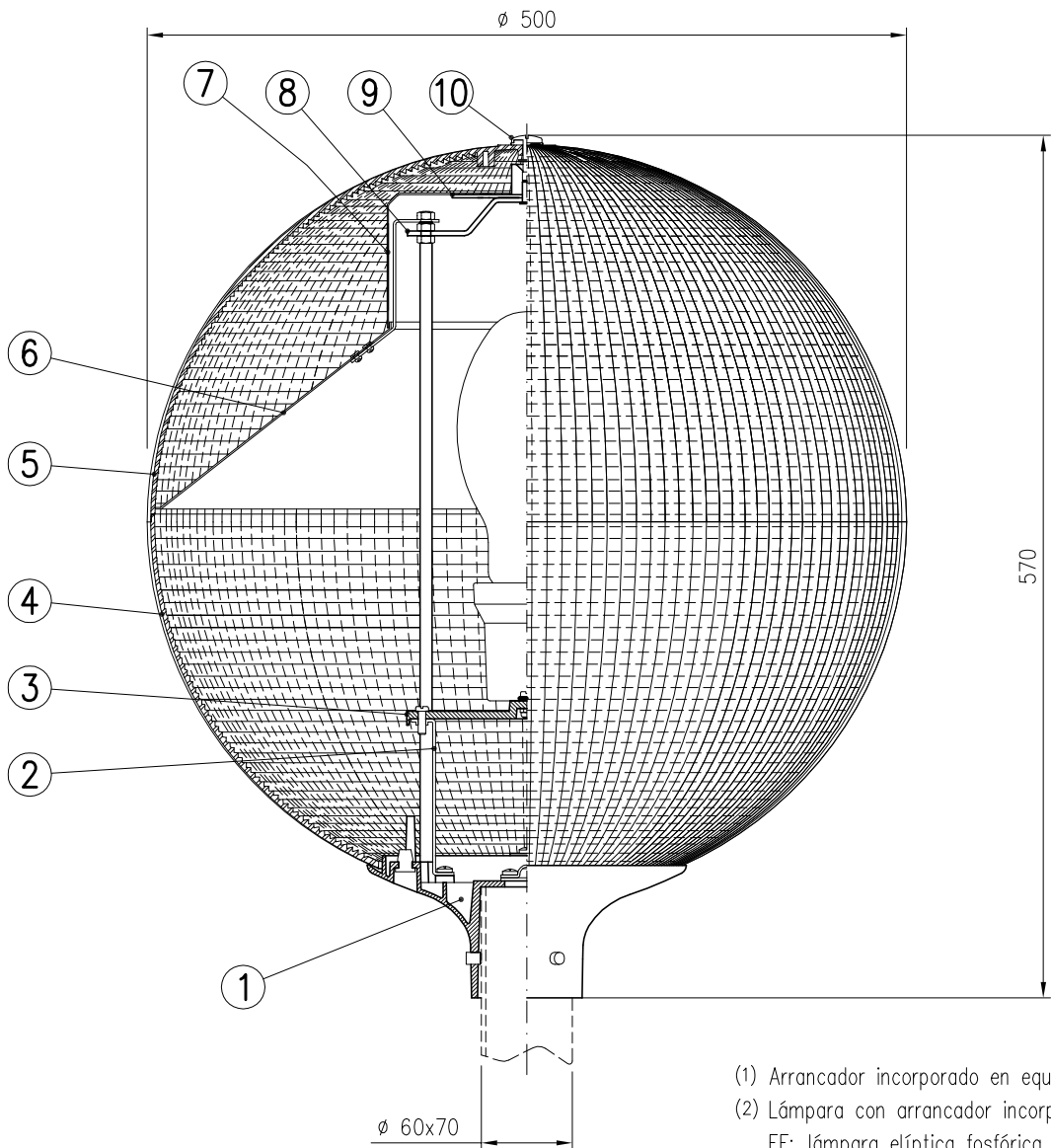
SEMI-SECCION LONGITUDINAL
