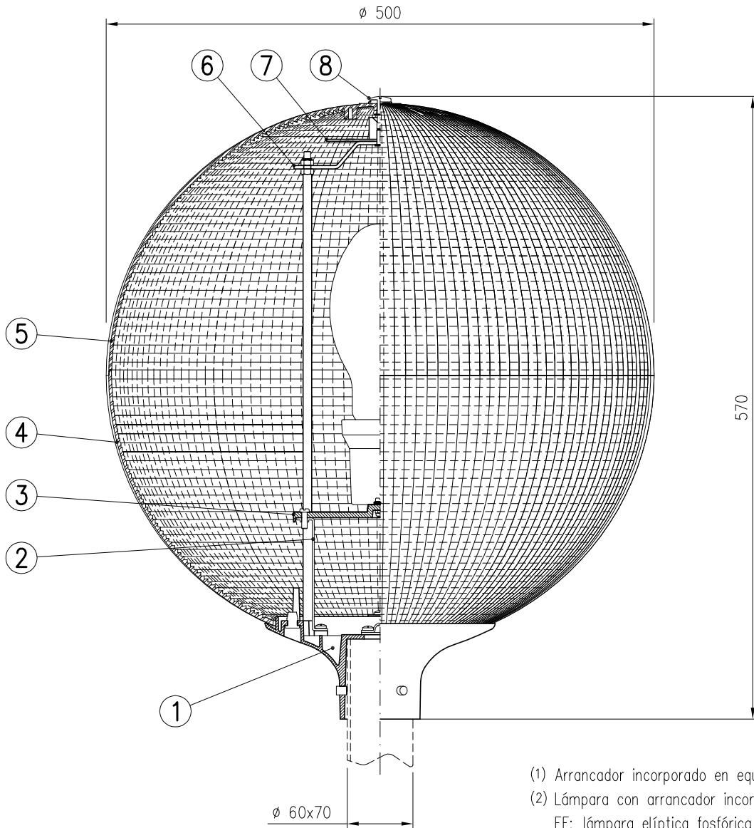
SEMI-SECCION LONGITUDINAL
