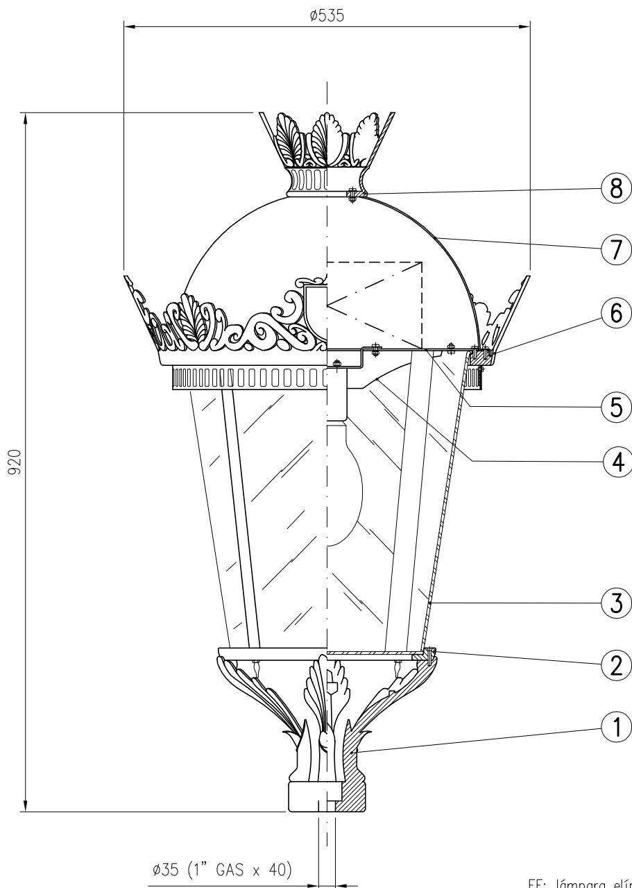
SEMI-SECCION LONGITUDINAL
