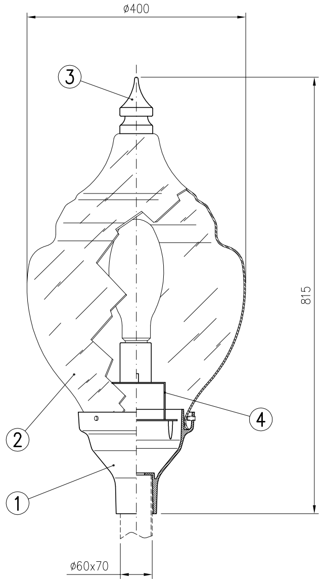
SEMI-SECCION LONGITUDINAL
