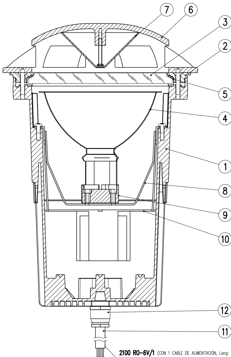
SECCION LONGITUDINAL
