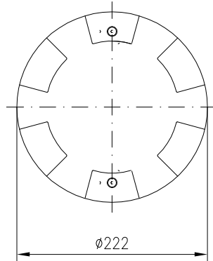
PLANTA
